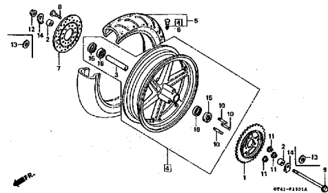
F-13-1 リヤーホイール (NSR50P・R・S) 114
