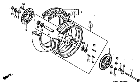
F-13 リヤーホイール (NSR50H・J・K・L・N) 112
