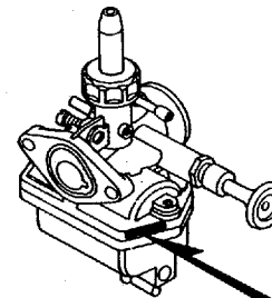
DGT4-B キャブレター号機打刻位置
