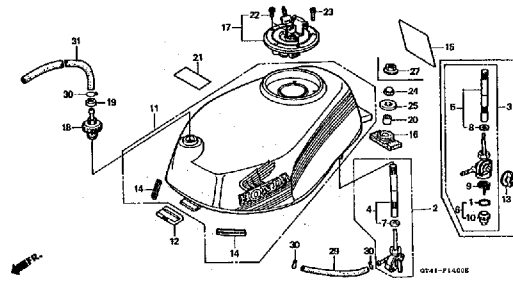
F-14 フューエルタンク 116
