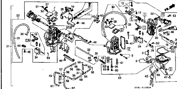
E-13 キャブレター F8
