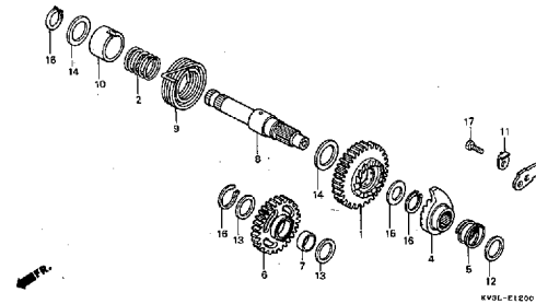
E-12 キックスタータースピンドル F7
